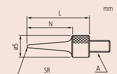
Jehlový dotek
