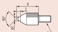
Kuželový dotek tvrdokovový (120057D)
