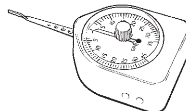
Zátěžový kalibr
