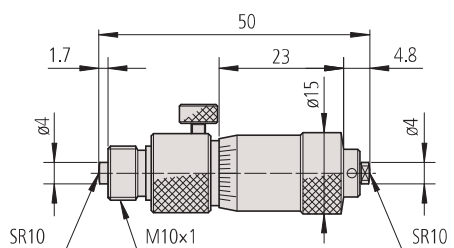
Mikrometrická hlava pro sérii 137
