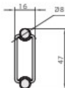
CARBON BAR SECTION SEZIONE ASTA IN CARBONIO
