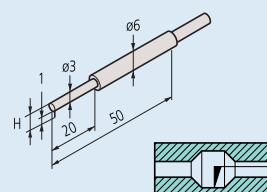
Pro malé otvory: 932694 / 12AAE874 Tvar hrotu: Jednostranně zkosžený / Kuželový Úhel hrotu: 20° / 30° Rádus hrotu: 25 µm / 25 µm Materiál hrotu: Tvrdokov / Tvrdokov
