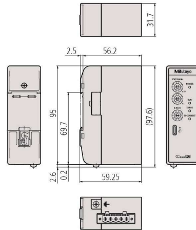
Jednotka rozhraní CC-Link (21HZA186)
