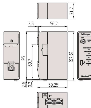
Jednotka rozhraní EtherNet/IP (21HZA188)
