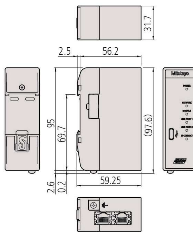
Jednotka rozhraní PROFINET (21HZA187)
