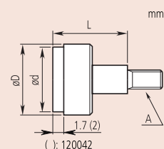
Plochý dotek - tvrdokovový (120041D)
