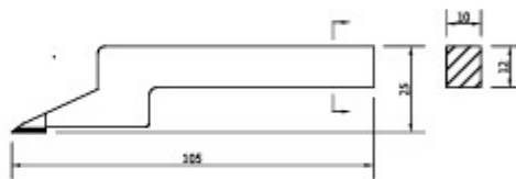
● 3130-4125 For:3130-8125 Range:0-600/0-24"
